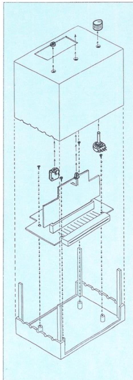
Figura 6. Inserimento del circuito nel contenitore.
